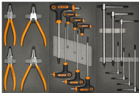
1815.150
