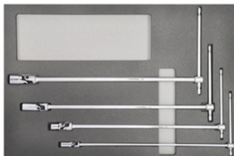
1815.380
